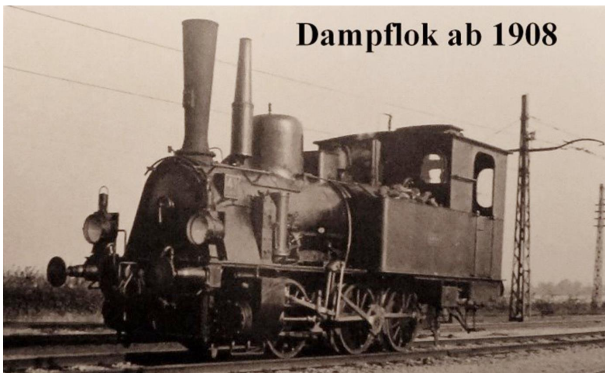
Der Einsatz von Dampflokomotiven wurde bis 1960 beibehalten. Lok 2b Humboldt, 1908.
